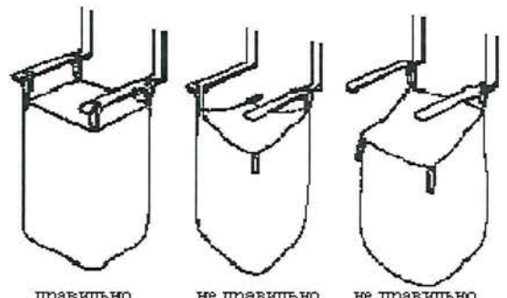
Рис. 8. Захват строп МК вилами погрузчика
