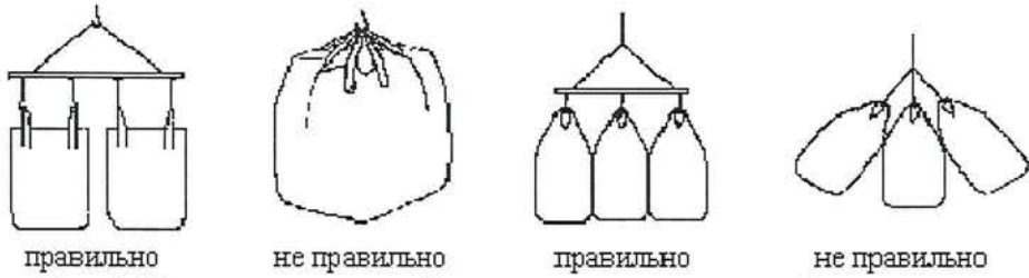
Рис. 4. Подъем мягких контейнеров с помощью крана, лебедки, тали.
